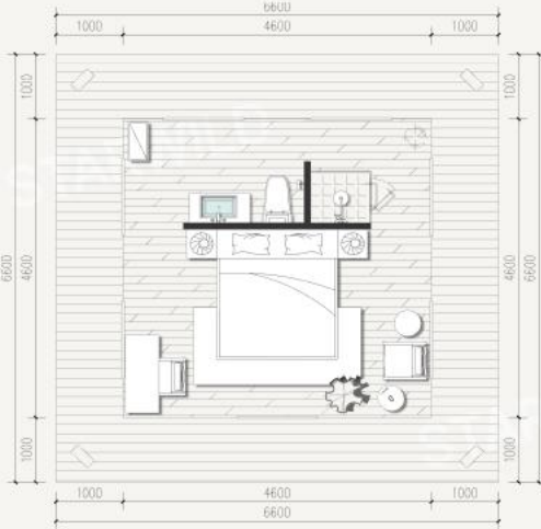
(6*6m Floor Plan)
